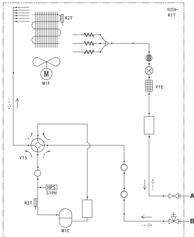
Legenda diagrama cevovoda
