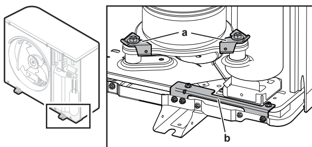
a Transportni varovali (2x) in podložki (2x)
